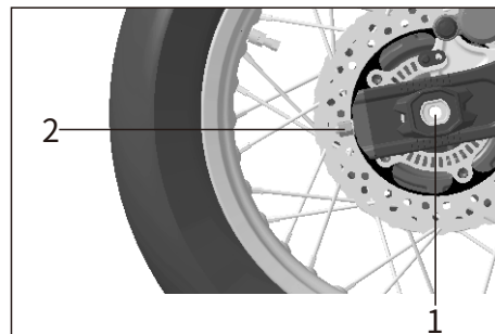
Couple de serrage de l'écrou de réglage : 14NM Couple de serrage de l'axe de roue arrière : 95NM
