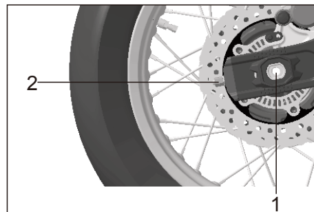
Couple de serrage de l'écrou de réglage : 22NM Couple de serrage de l'axe de roue arrière : 95NM
